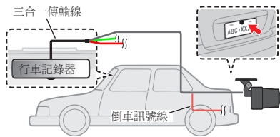
車外型後鏡頭安裝示意圖
